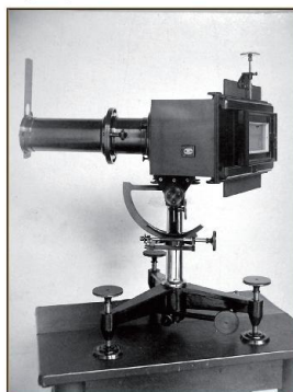
A Konkoly Thege által kifejlesztett spektrográf az egész világon elterjedt
